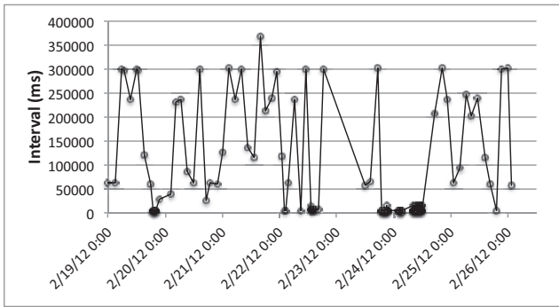
Fig. 7. Feed 504.1, update interval
