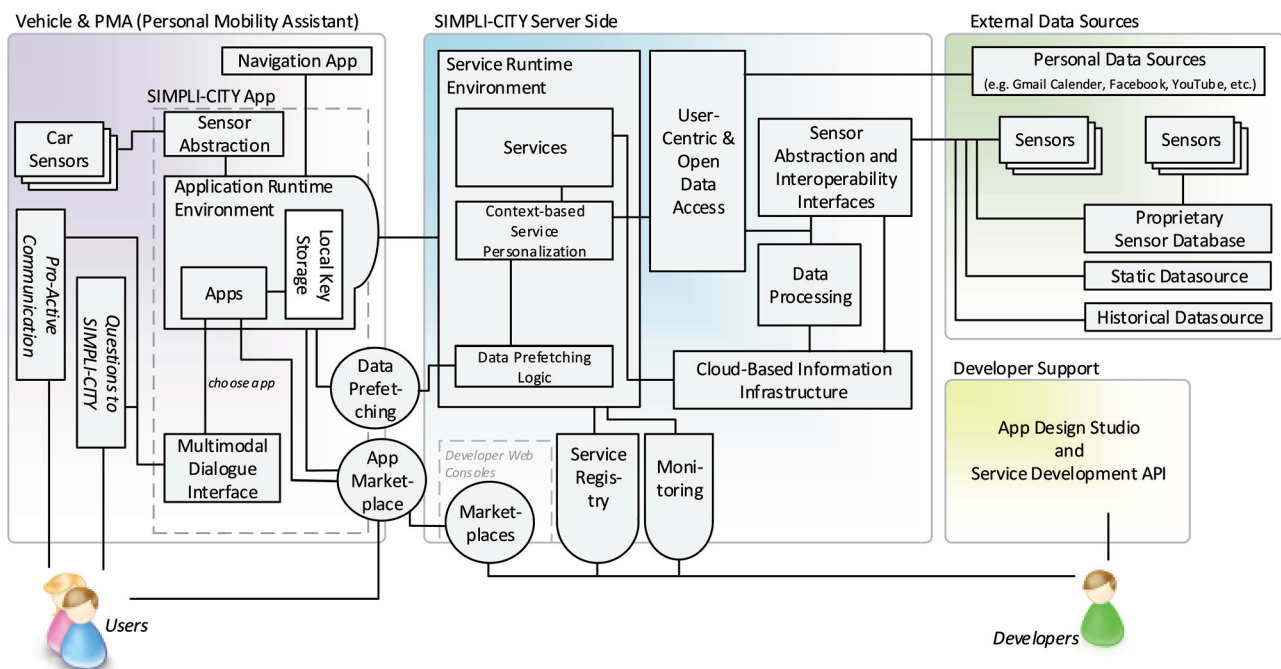
Abbildung 1: SIMPLI-CITY-Gesamtarchitektur
